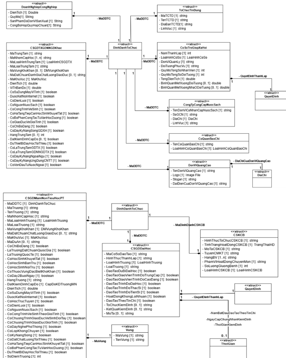
Hình A.2.7. Cấu trúc và mối quan hệ giữa các cấu trúc trong mô hình dữ liệu pháp nhân được mô tả bằng ngôn ngữ UML - Hoạt động trong các lĩnh vực
