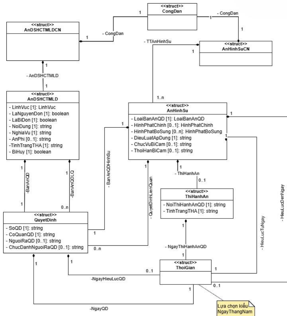
Hình A.1.10. Cấu trúc và mối quan hệ giữa các cấu trúc trong mô hình dữ liệu về con người được mô tả bằng ngôn ngữ UML - Các vấn đề liên quan đến pháp luật
